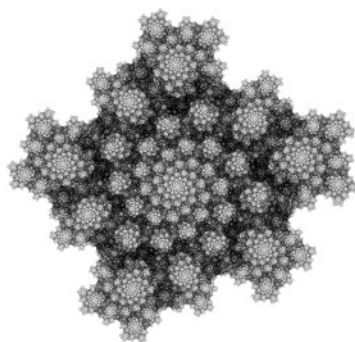
図2. ロマネスコとフラクタル( a_1=0.2044+0.9355i , a_2=-0.2262-0.291i )
