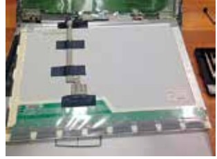
写真4. 液晶パネルを外す
