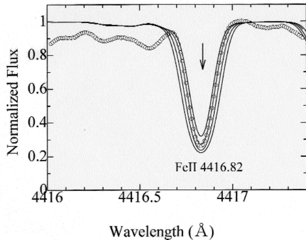
図1：HD 221568（大沢スター）に見られる一回電離鉄（Fe II 4416.82）の吸収線。白丸は観測（すばる望遠鏡/HDS）で得られたスペクトル。実線は上から1キロGauss，2キロGauss（青線），3キロGauss，4キロGaussを仮定したときに予想されるスペクトル。この場合、微視的乱流速度を0km/sとしました。鉄の組成比は太陽値の14倍と求まりました。
