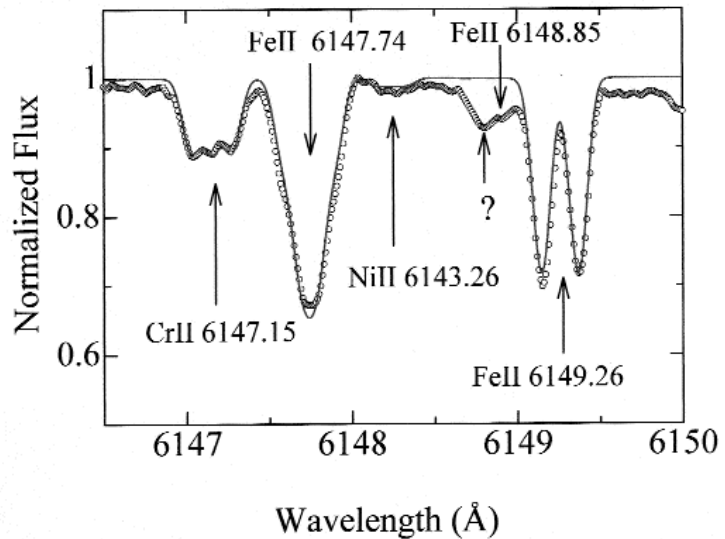
図 3 : HR 5049 のスペクトル。白丸は観測スペクトル (ESO EMMI), 青線は磁場の強さを 4.7 キロガウスとした時の合成スペクトル。一回電離鉄 (FeII 6149.26) はゼーマン効果により 2 本に分岐しています。モデル大気の有効温度を 11000K, 表面重力加速度 ( \log g ) を 4.0 としたとき、鉄の組成比は太陽値の 10 倍、クロムは 166 倍となり、10300K, 3.8 の値は鉄が 7.4 倍、クロムが 120 倍となりました。
