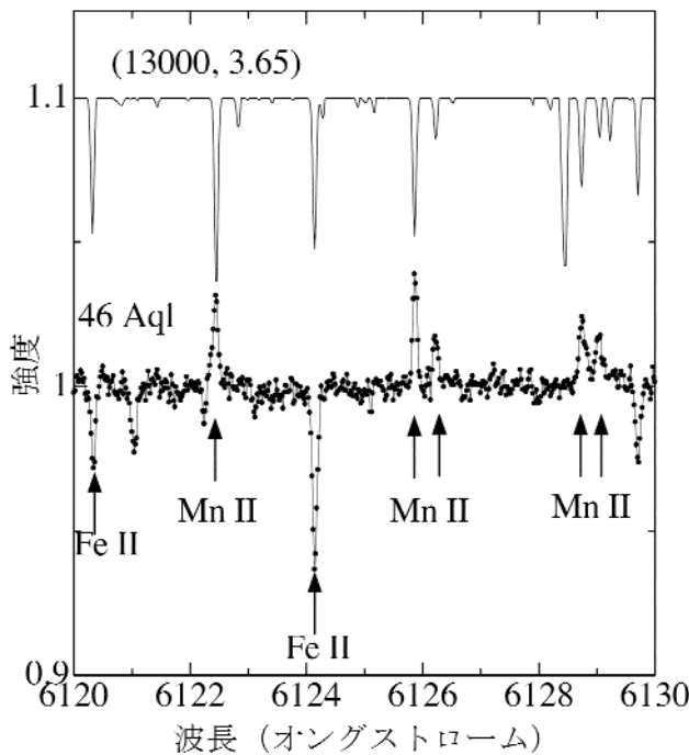
図4：46 Aql (HD 186122)に見られる一回電離マンガン(Mn II)の輝線。細実線は、有効温度 13,000 K、表面重力加速度(log g) 3.65 の大気モデルで予想されるスペクトル。一回電離鉄(Fe II)の線は予想通り吸収線になっていますが、Mn II の線は全部輝線として見えています。すばる望遠鏡(HDS) で得られたデータです。
