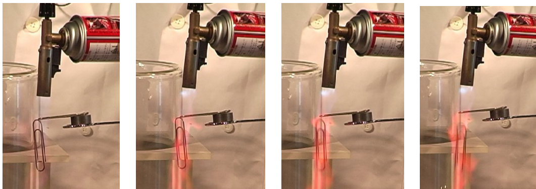
図1 熱い鉄が磁石に反応しないことを確かめる実験。中央の黒い塊がフェライト磁石。これにクリップをつけて、その先に別のクリップを磁力で吊るして、クリップを熱する。
