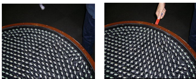
図4 方位磁石結晶（左）に棒磁石を近づけると多くの方位磁石が磁石と同じ向きになる（右）。
